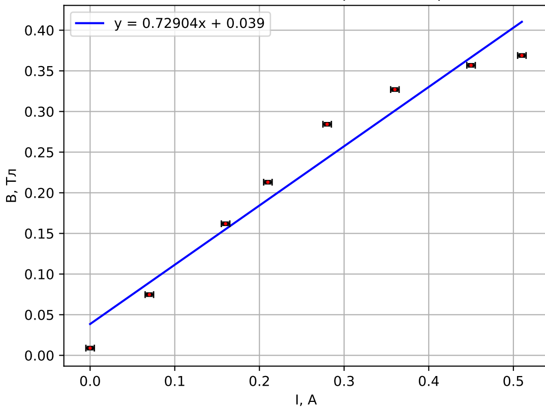
Зависимость В от I (калибровочная кривая)
